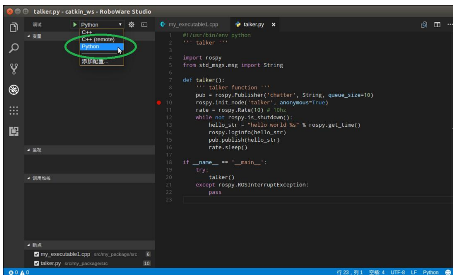
图 3-23 在调试视图中, 将调试器设置为“Python”
