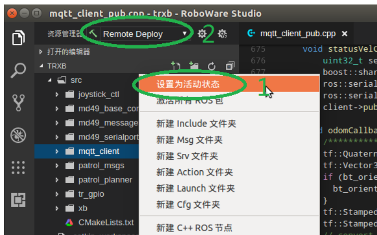
图 3-40 远程部署一个或多个包
