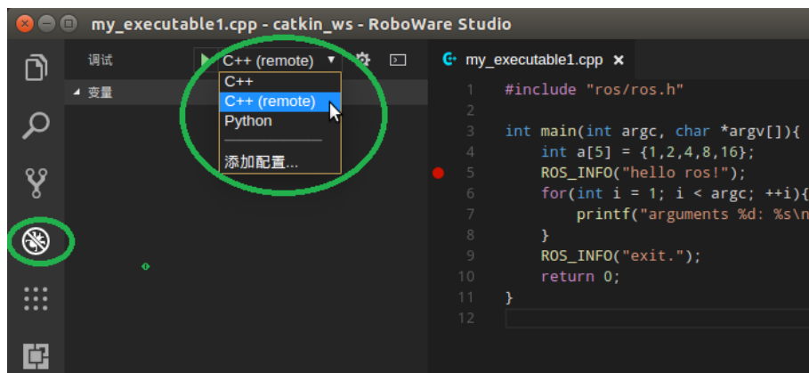
图 3-38 在调试视图下，调试器自动设置为“C++ (remote)”
