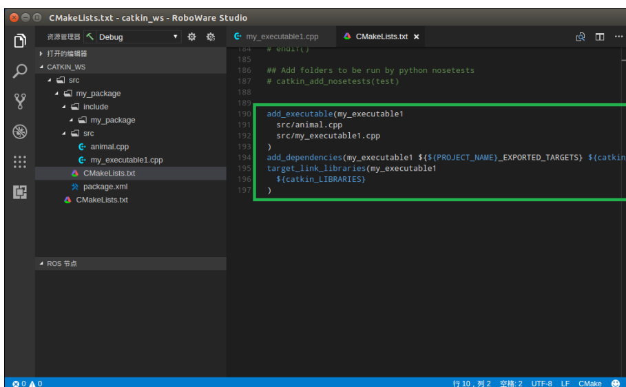
图 3-7 CMakeLists.txt 文件自动更新
