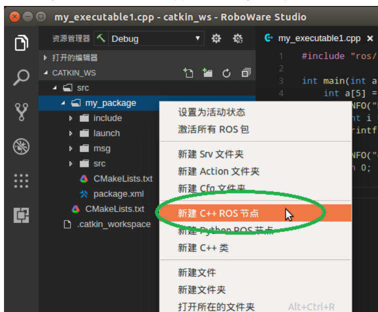
图 3-44 节点、类创建向导
