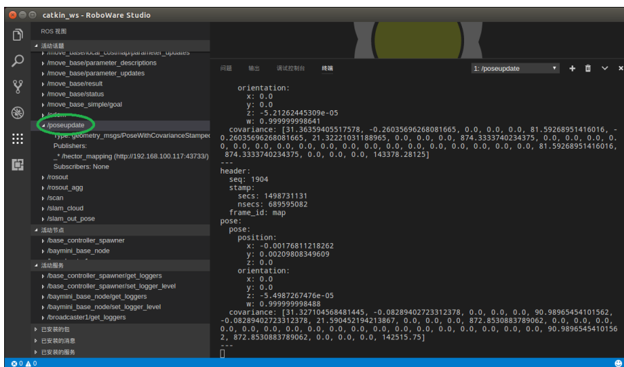
图 3-51 双击查看话题的实时数据流
