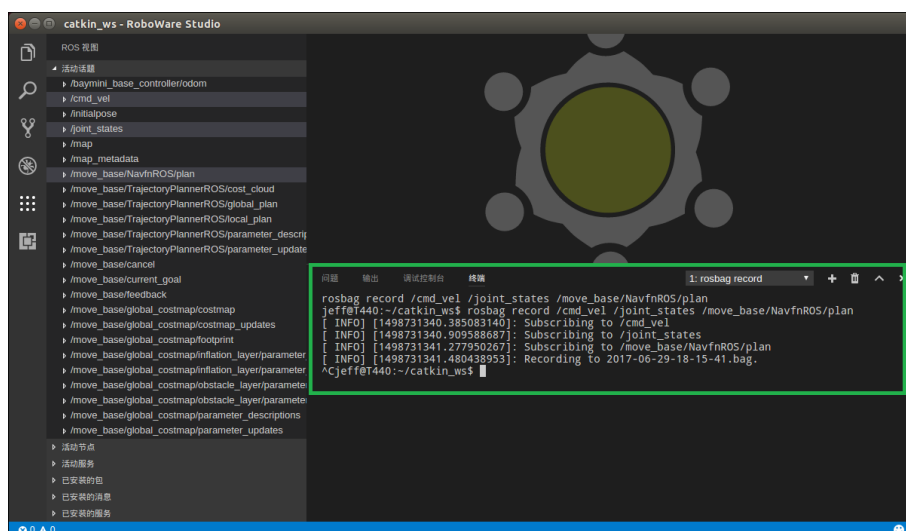
在集成终端按“Ctrl+c”停止记录
