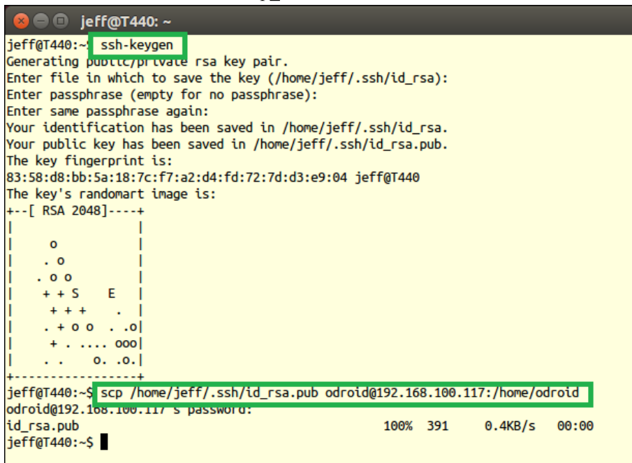
图 3-30 在本地计算机生成密钥，并将公钥文件拷贝到远程计算机
