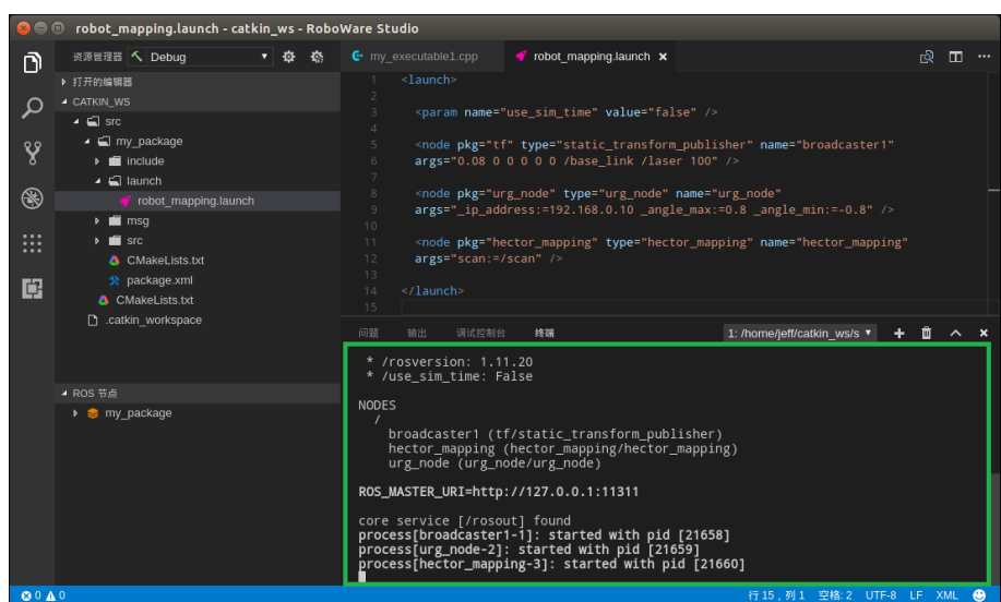
图 3-28 launch 文件在集成终端中运行
