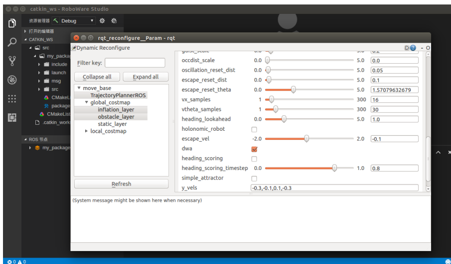
图 3-48 启动 rqt-reconfigure
